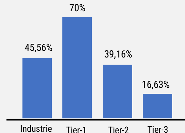
Gesamt-THG-Emissionen
