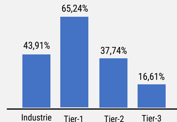
CO 2 - Fußabdruck
